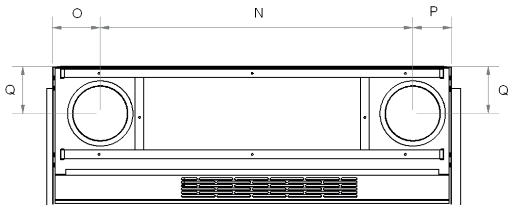
Abb. 9 Platzierung der Durchführungen
