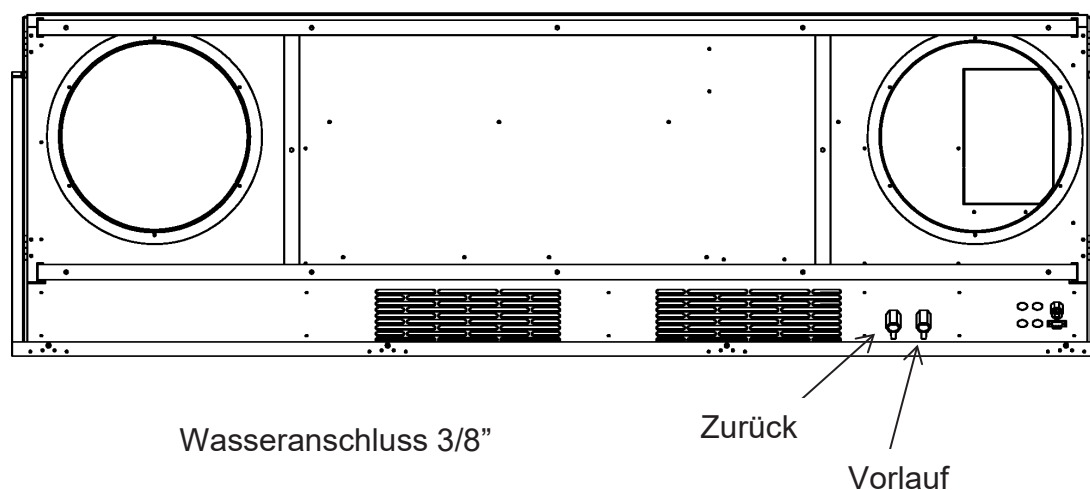
Abb. 11 Wasseranschluss
