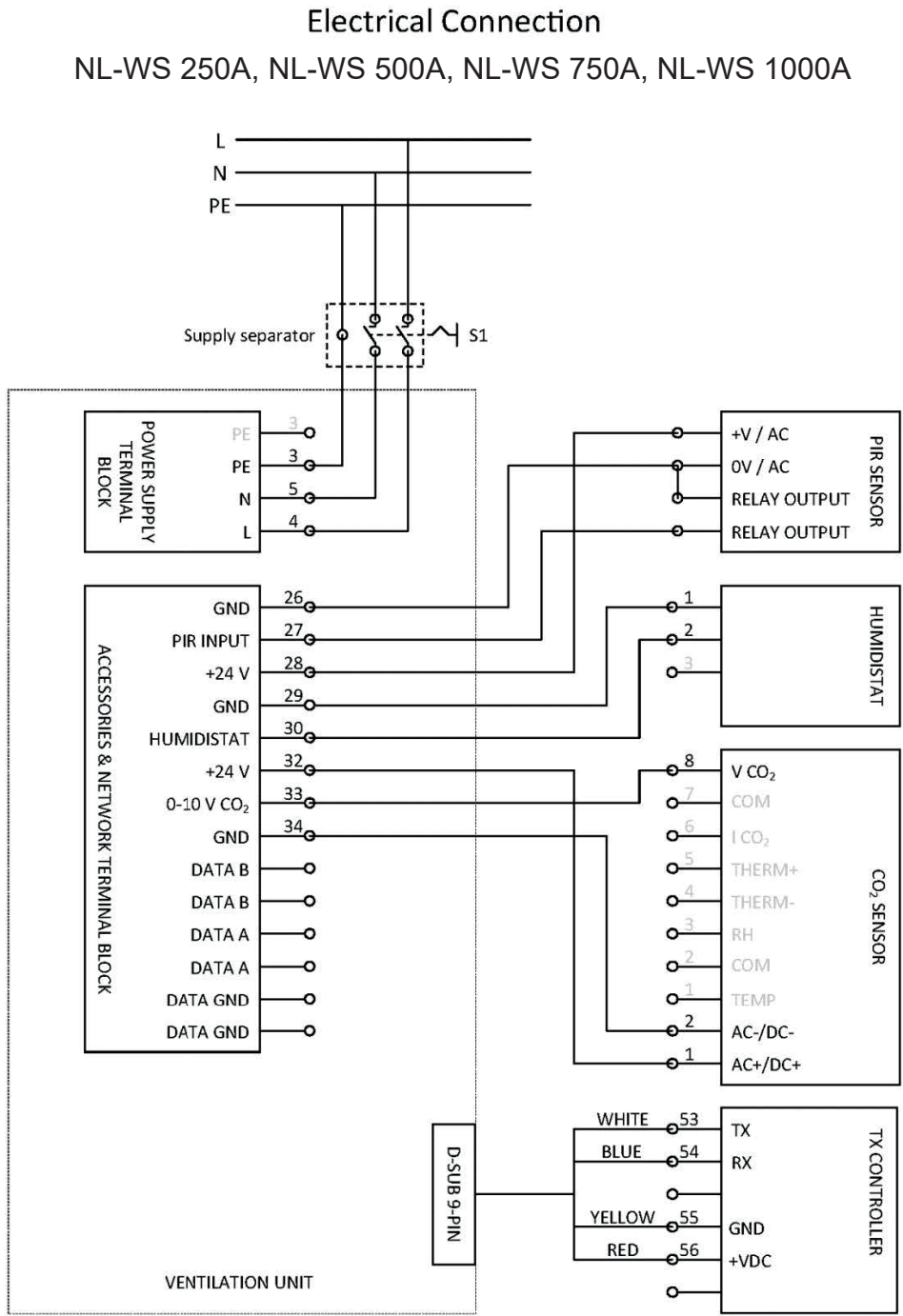
Abb. 13 Elektroschaltplan für Zubehör
