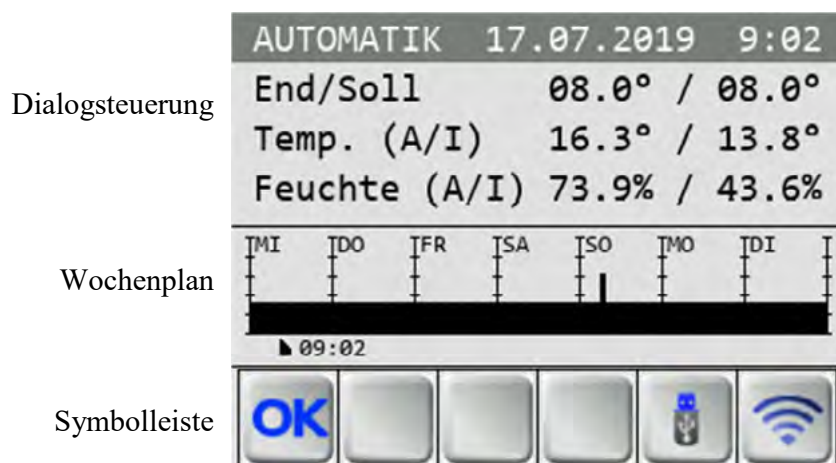
Abbildung 2) Typische Darstellung der Aufheizautomatik
