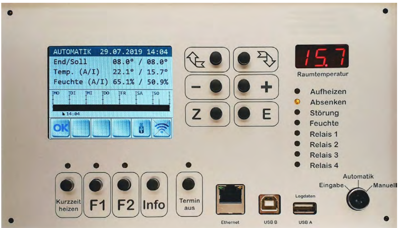
Abbildung 1) Bedienoberfläche der Kirchengaufheizautomatik
